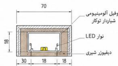
دیتیل نور مخفی Sc:1/5
