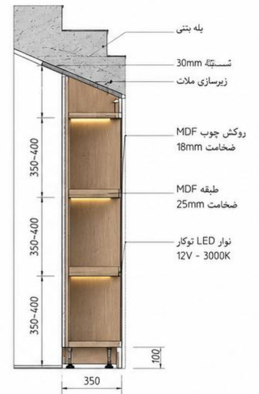
برش A-A Sc:1/20
